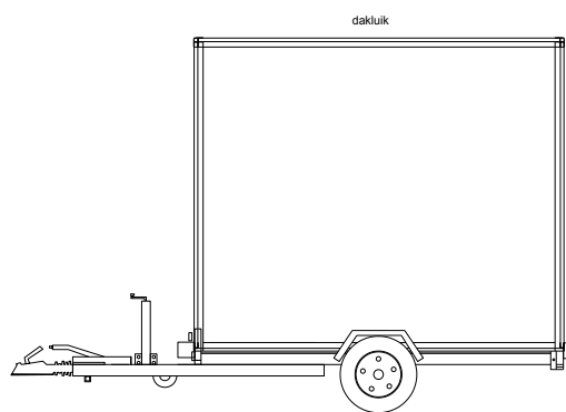
Linkeraanzicht
