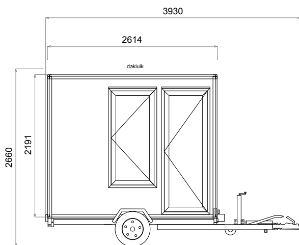
Linkeraanzicht
